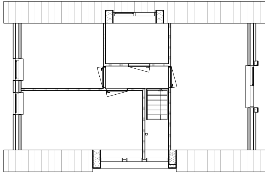
eerste verdieping optie gevel variant 2 optie dakkapel
