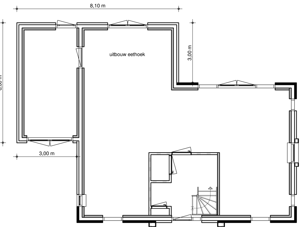
begane grond optie uitbouw eethoek
