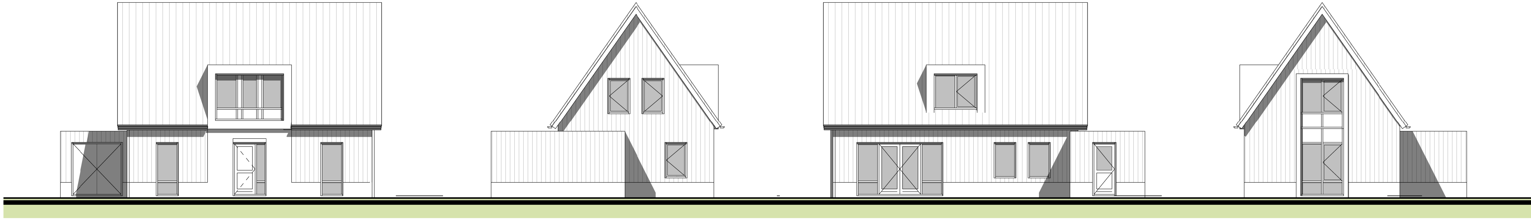
voorgevel optie gevel variant 2
