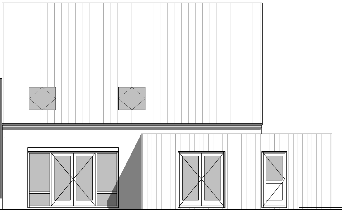
achtergevel optie uitbouw eethoek
