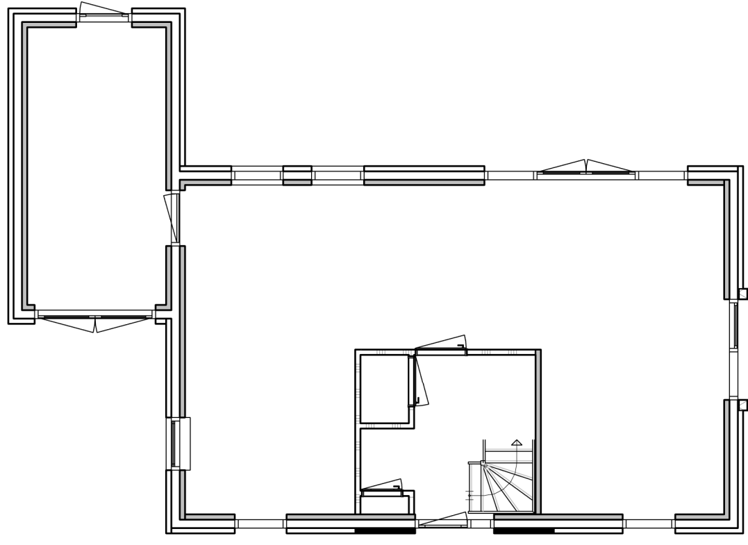
begane grond optie gevel variant 2
