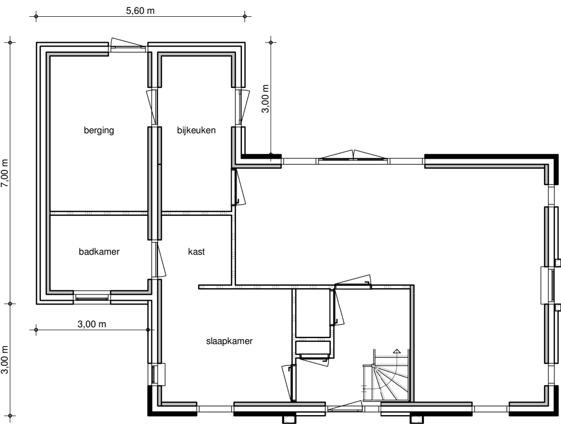
begane grond optie slaapkamer en badkamer optie bijkeuken
