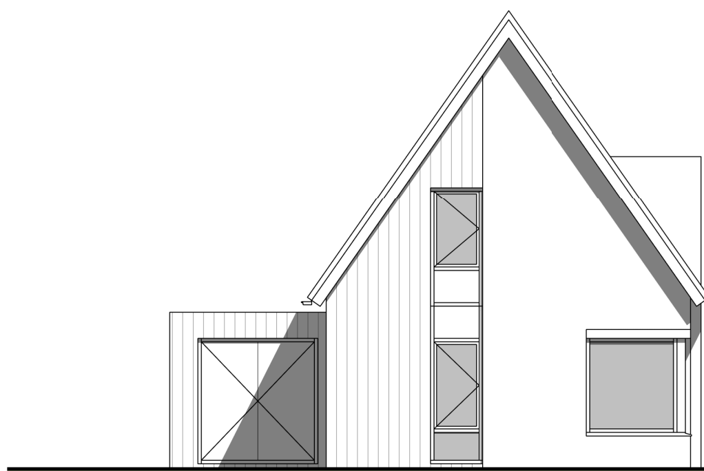
voorgevel optie entree in zijgevel
