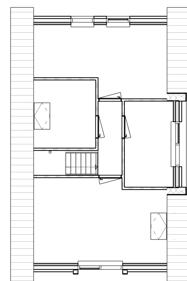
eerste verdieping optie gevel variant 2
