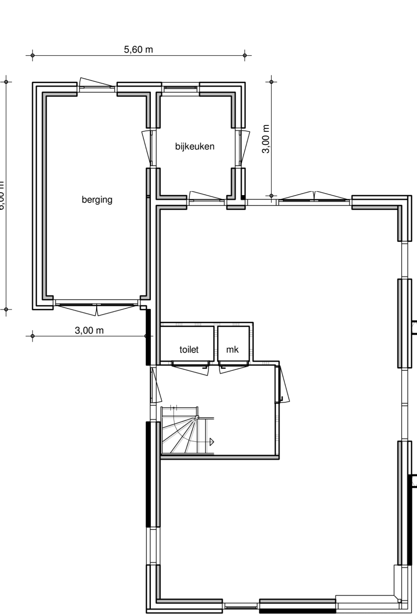
begane grond optie entree in zijgevel
