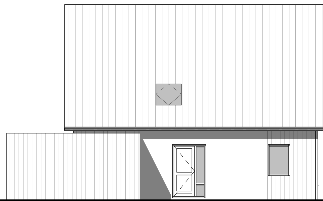
linkergevel optie entree in zijgevel
