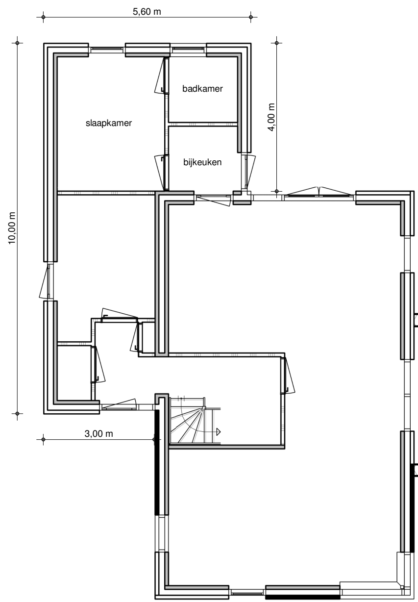
begane grond optie slaapkamer en badkamer
