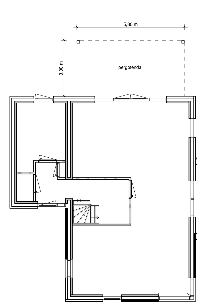
begane grond optie pergotenda
